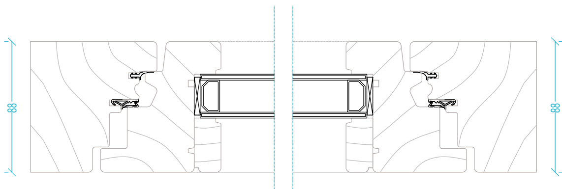
Sezione orizzontale
