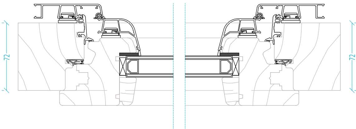
Sezione orizzontale
