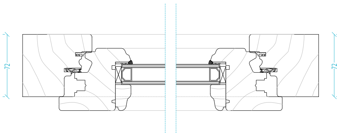
Sezione orizzontale
