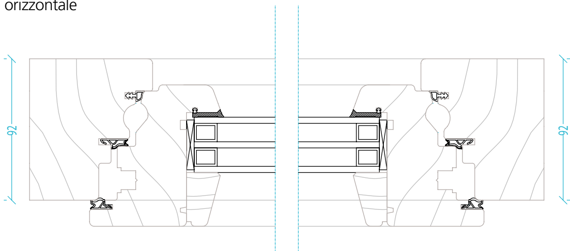
Sezione orizzontale
