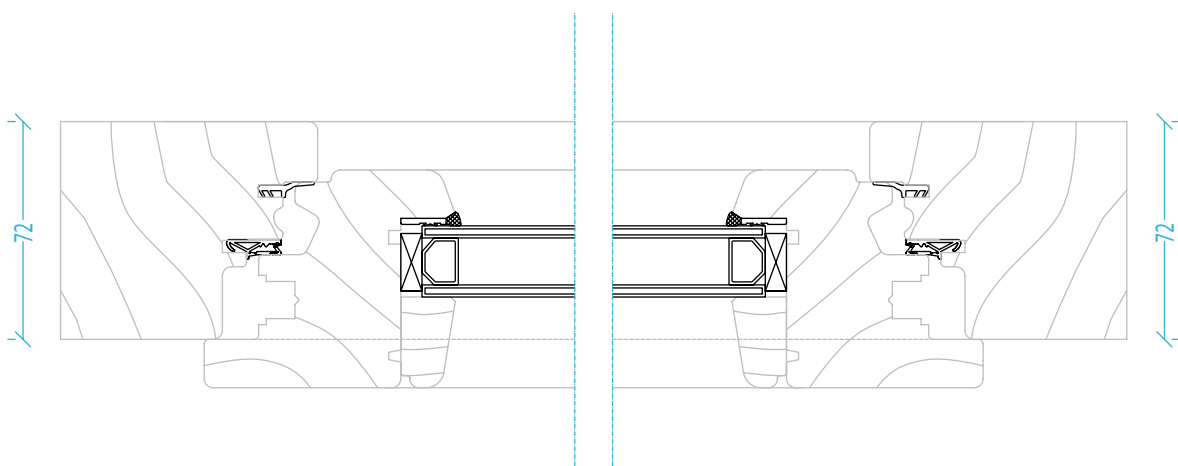
Sezione orizzontale
