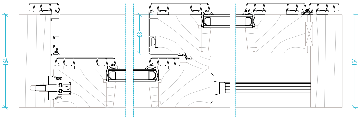
Sezione orizzontale
