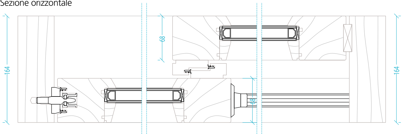
Sezione orizzontale
